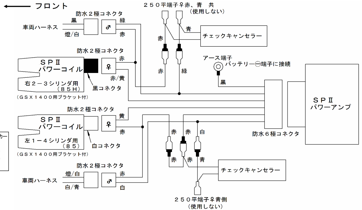
図2 配線図
