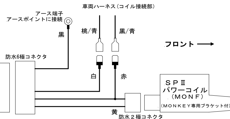
図1配線図
