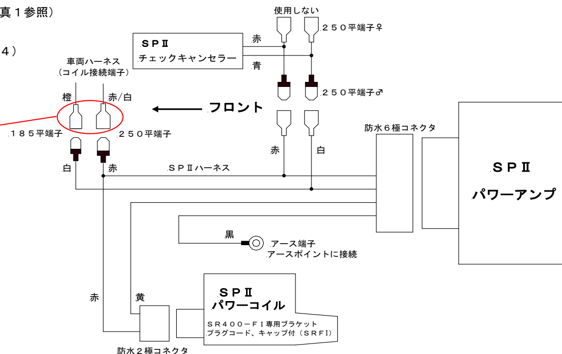
図1配線図
