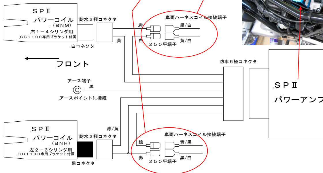
図2配線図
