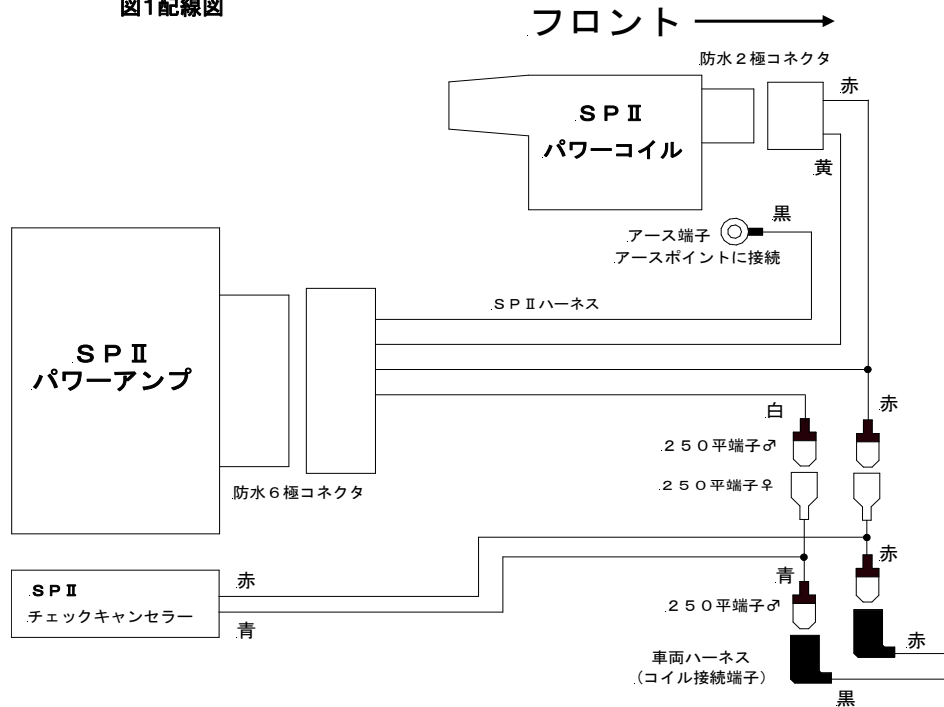
図1配線図
