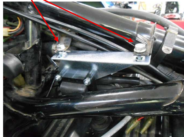
図2、左側コイル
