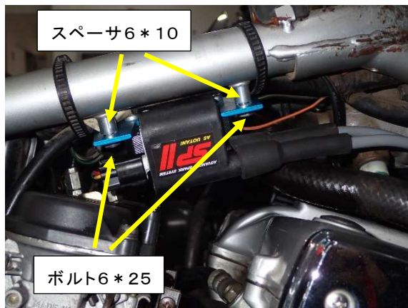
図3、#1&4コイル
