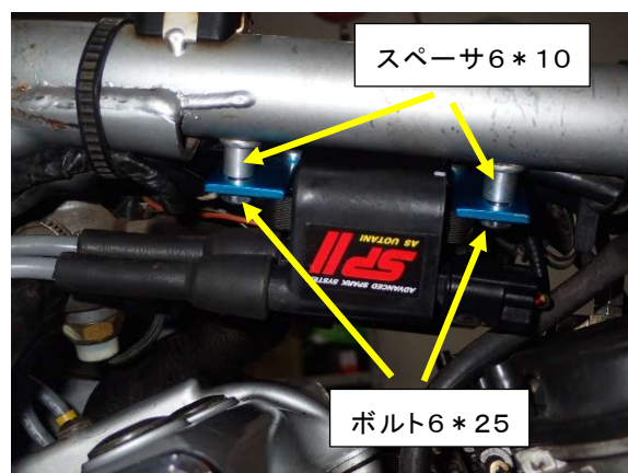
図4、#2&3コイル
