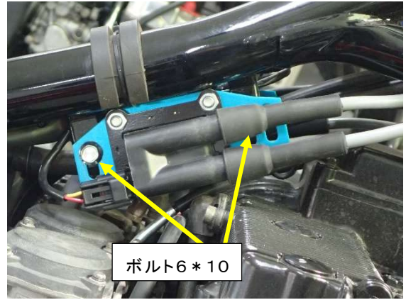
図4、#2&3コイル
